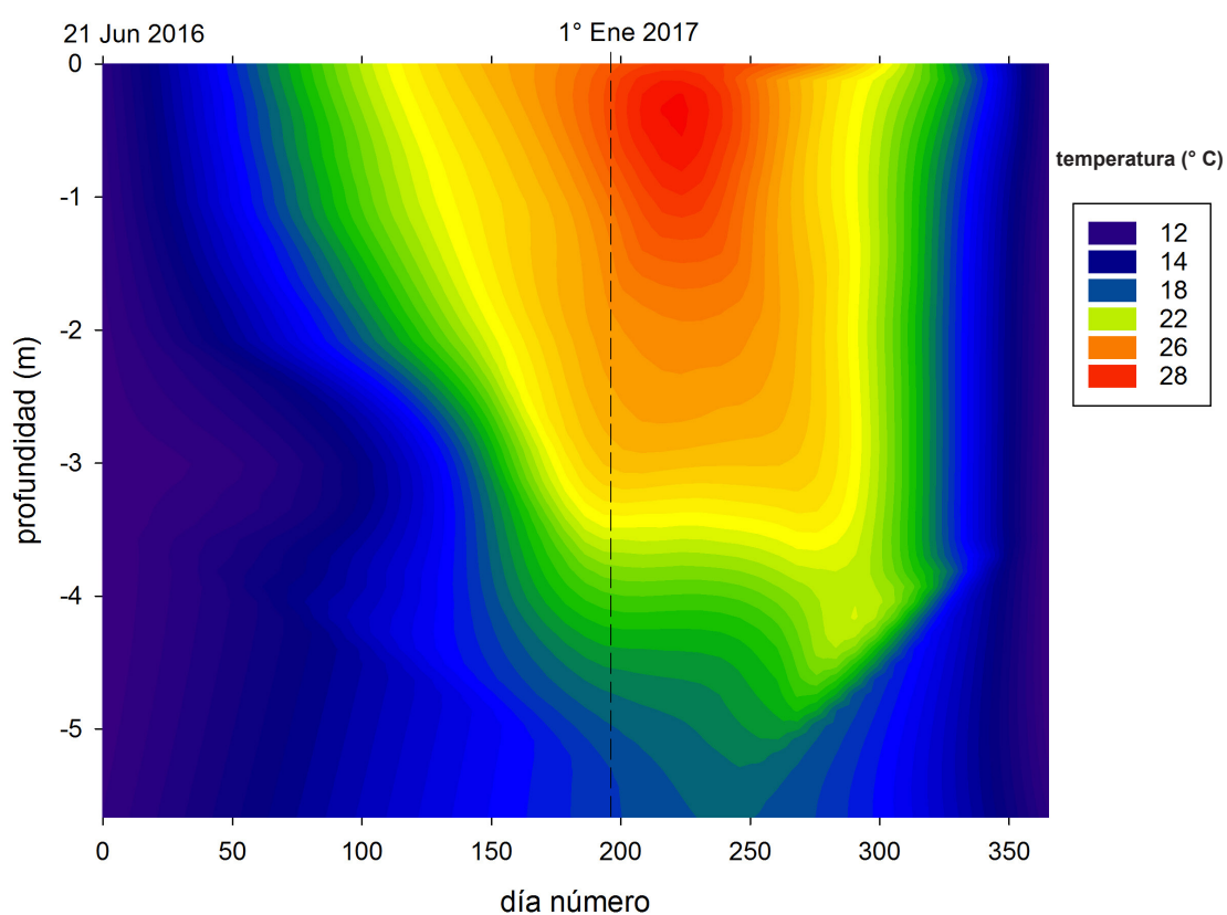
Variación de la temperatura del agua con la profundidad, para el período junio 2016-junio 2017. Lago Jardín de Lagomar. Obsérvese como la diferencia vertical de temperatura es intensa en verano e inexistente en invierno.
